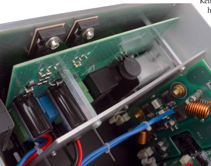
Eines der Geheimnisse der Endstufe ist der „Cap Multiplier“, der elektronisch große Siebkapazitäten nachbildet
